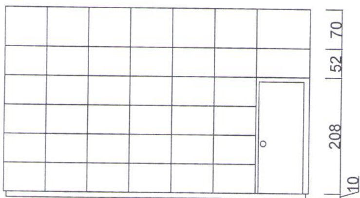
CORTE BB
