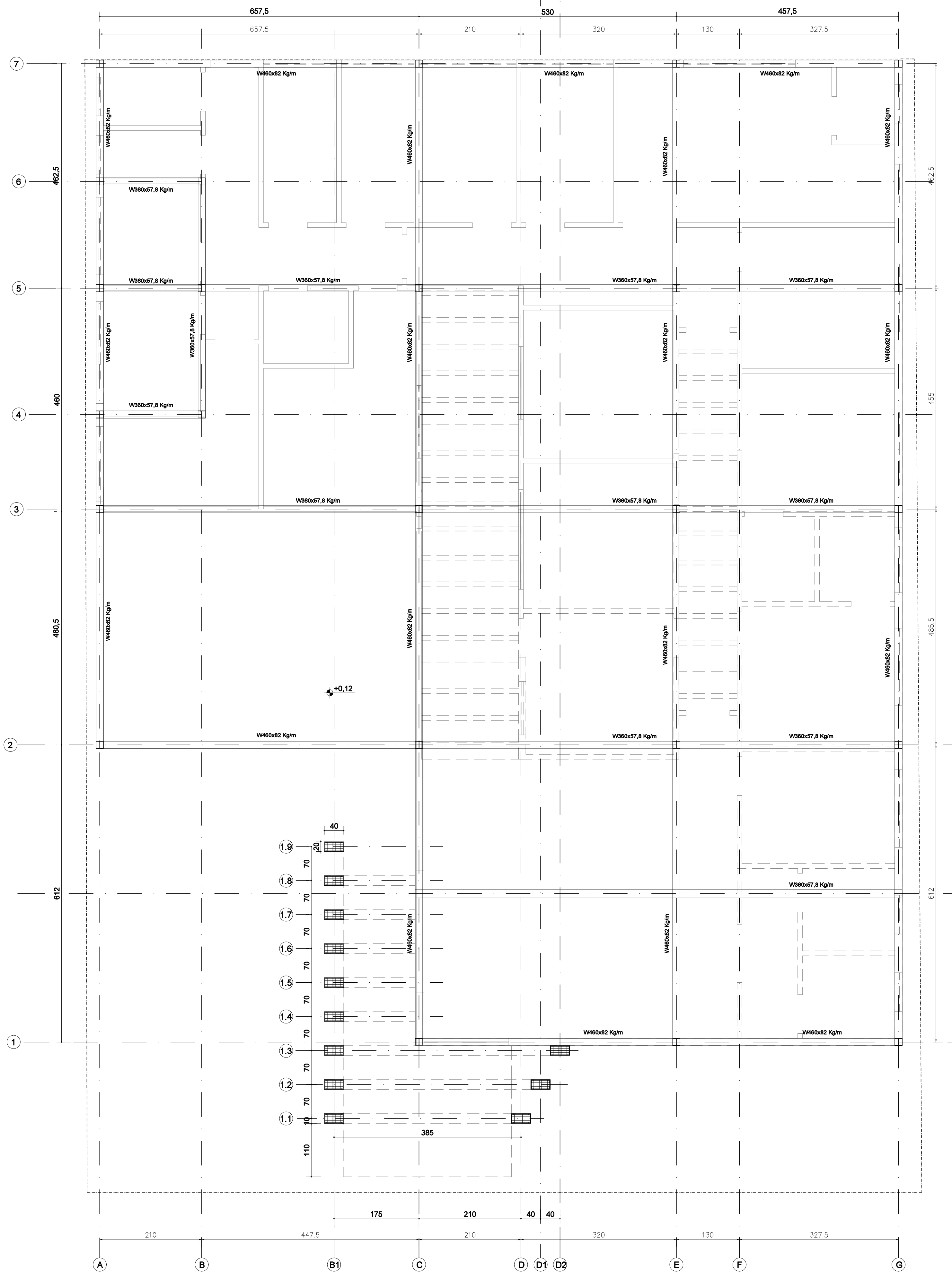
PLANTA NÍVEL +0,12 ESCALA 1/50
